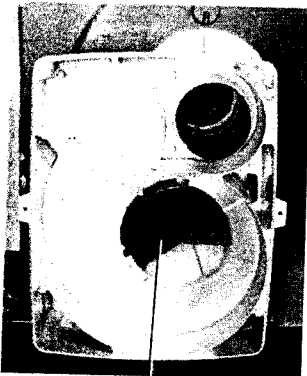
Ansaugluftführung
