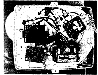
Einbaulage Brenner bei NU-3-40/-50 und HU-5-37/-45
