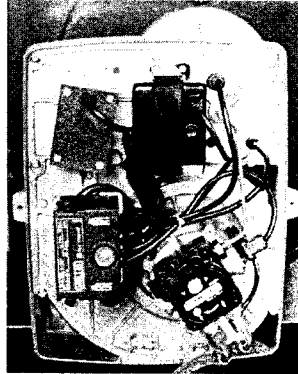
Einbaulage Brenner bei NU-3-17/-20/-25/-32 und HU-5-22/-29
