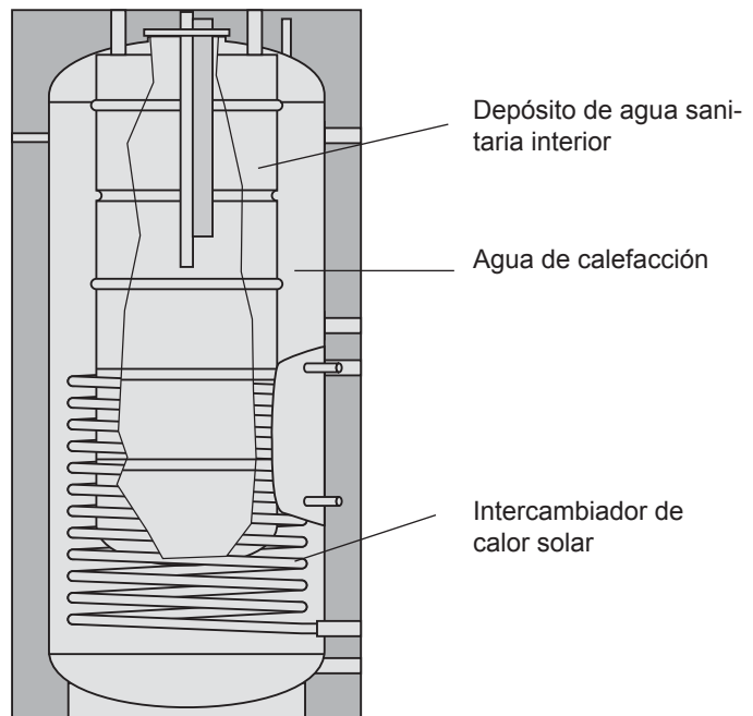
Acumulador doble SED-750/250
