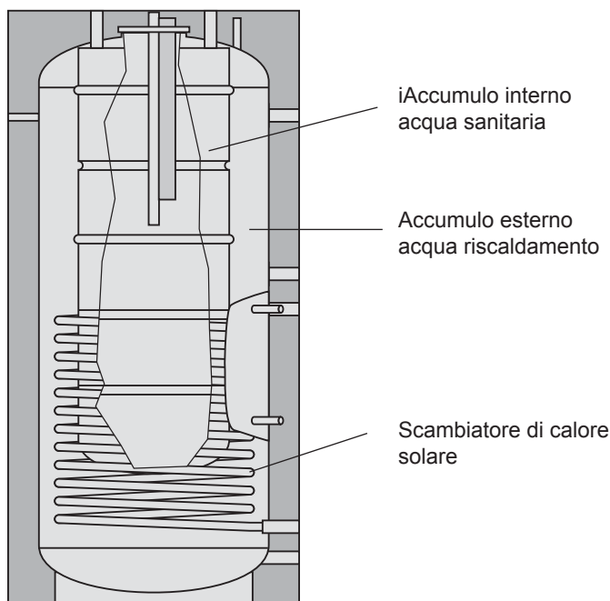
Bollitore doppio SED-750/250
