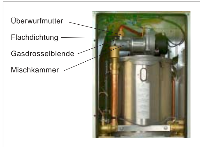
Bild 2: Bauteile
