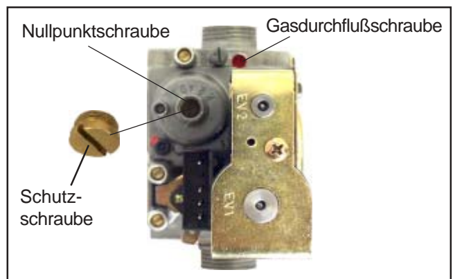
Bild: Gaskombiventil
