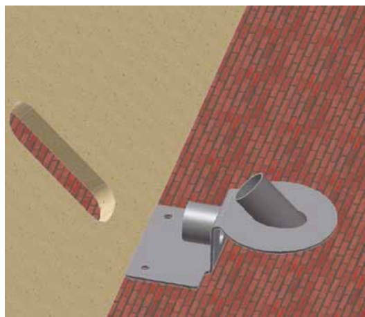
Abb. Nr.4 Variante 2: Saugpunkt am Boden montiert
